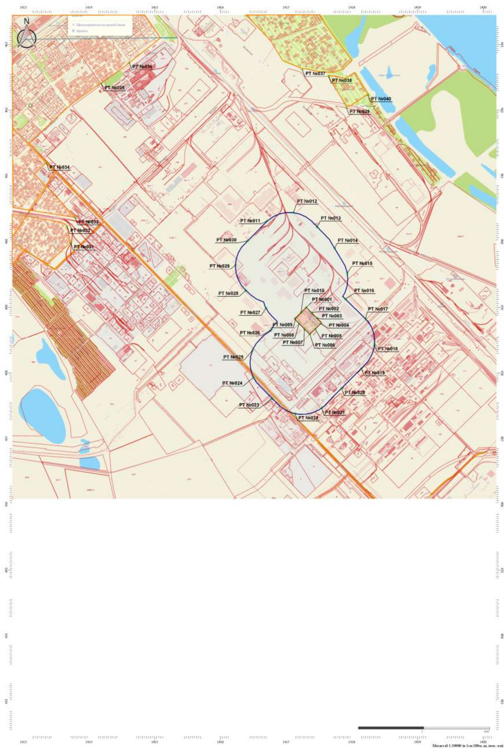
Рисунок 6.2 - Карта-схема расположения расчетных точек на период строительства
