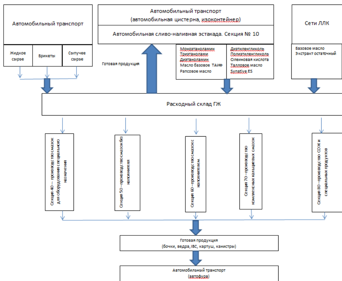
Рисунок 6.12 - Блок-схема основных технологических потоков с указанием наименования опасных веществ и направления их перемещения в технологической схеме
