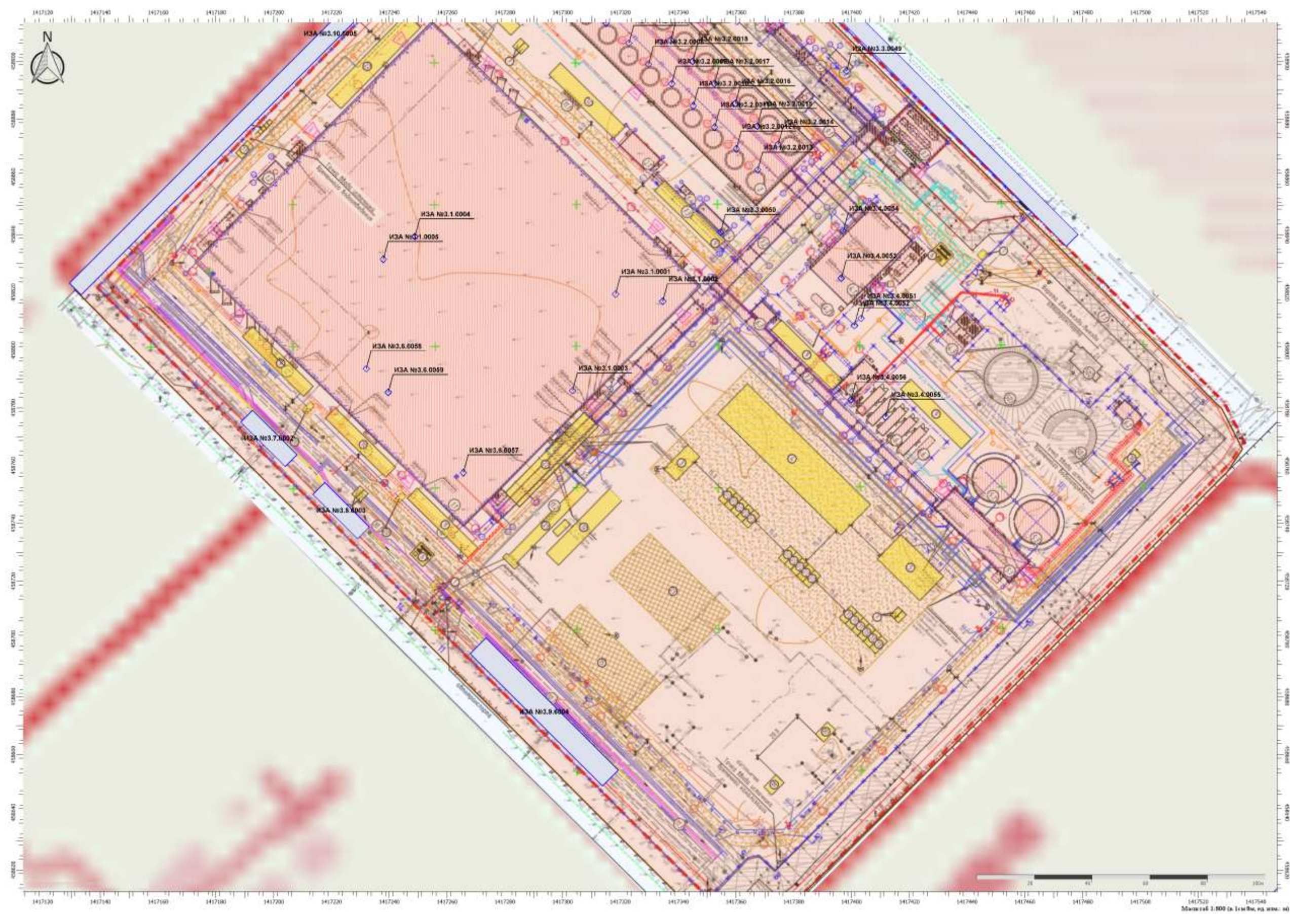
Рисунок 6.5. Лист 2 Карта-схема расположения источников выброса на период эксплуатации
