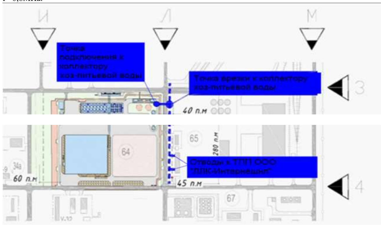
Рисунок 6.8 - Точка подключения к существующей сети хозяйственно-питьевого водоснабжения ООО «ЛУКОЙЛ-Волгограднефтепереработка»
