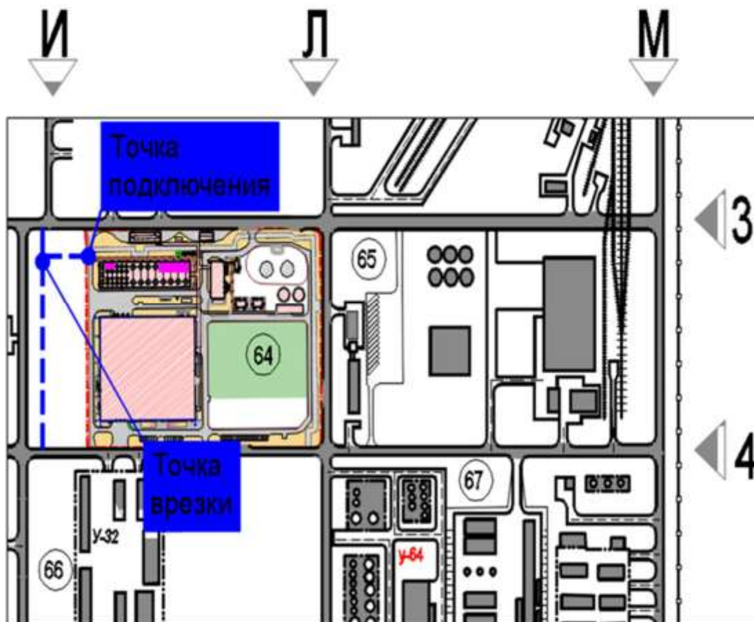
Рисунок 6.9 - Точка подключения к существующей сети технической (речной) воды ООО «ЛУКОЙЛ-Волгограднефтепереработка»
