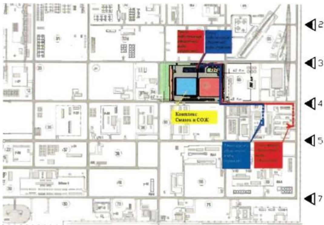
Рисунок 6.10 - Точка подключения к существующей сети оборотной воды ООО «ЛУКОЙЛ-Волгограднефтепереработка»
