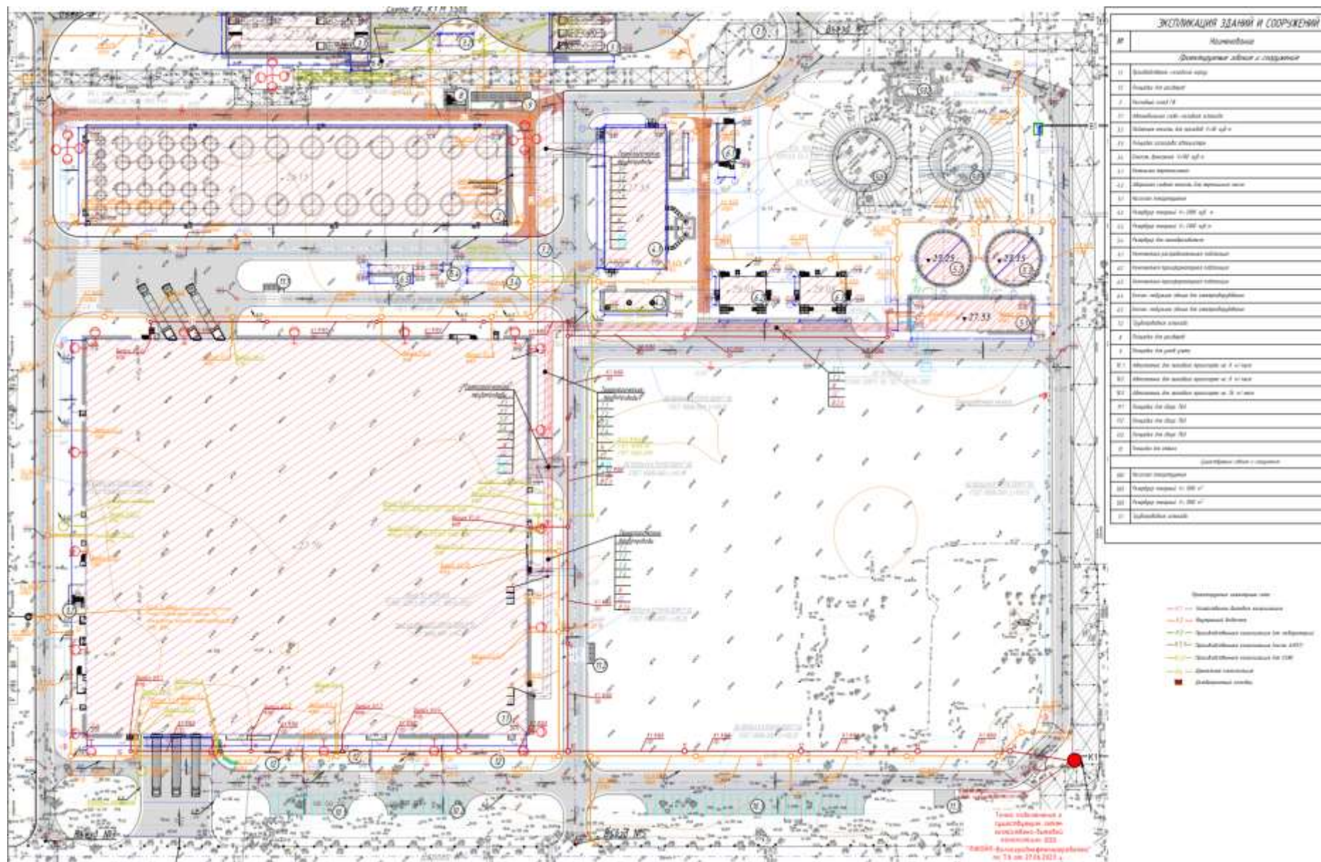
Рисунок 6.11 - Схема сетей канализации проектируемого объекта.
